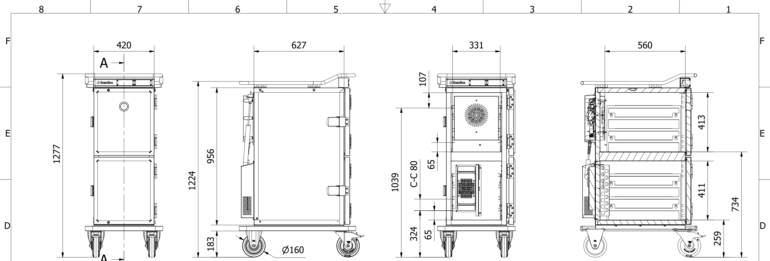
A-A ( 1:13 )
