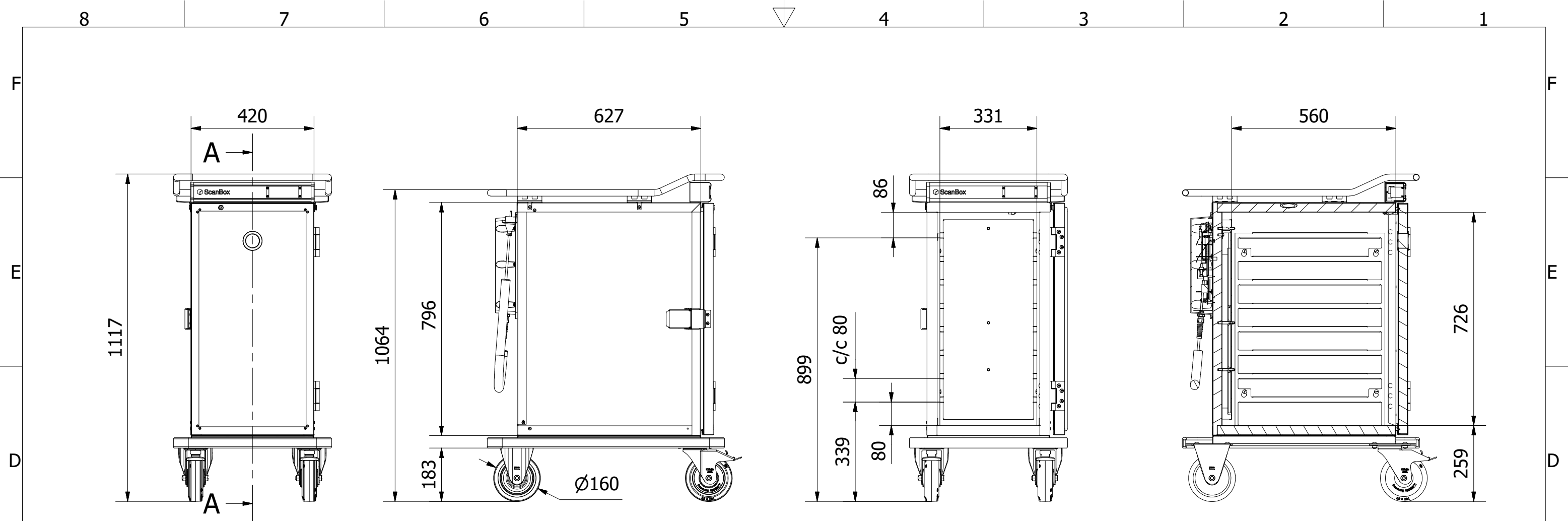
A-A ( 1:13 )
