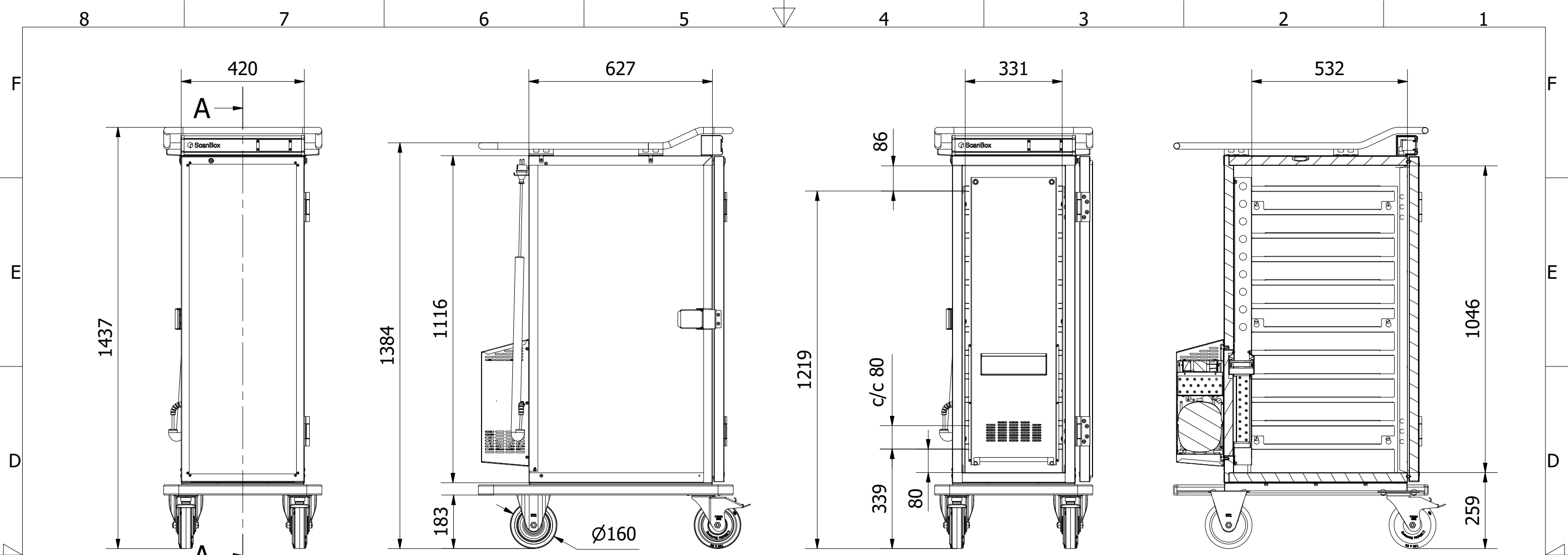
A-A ( 1:13 )
