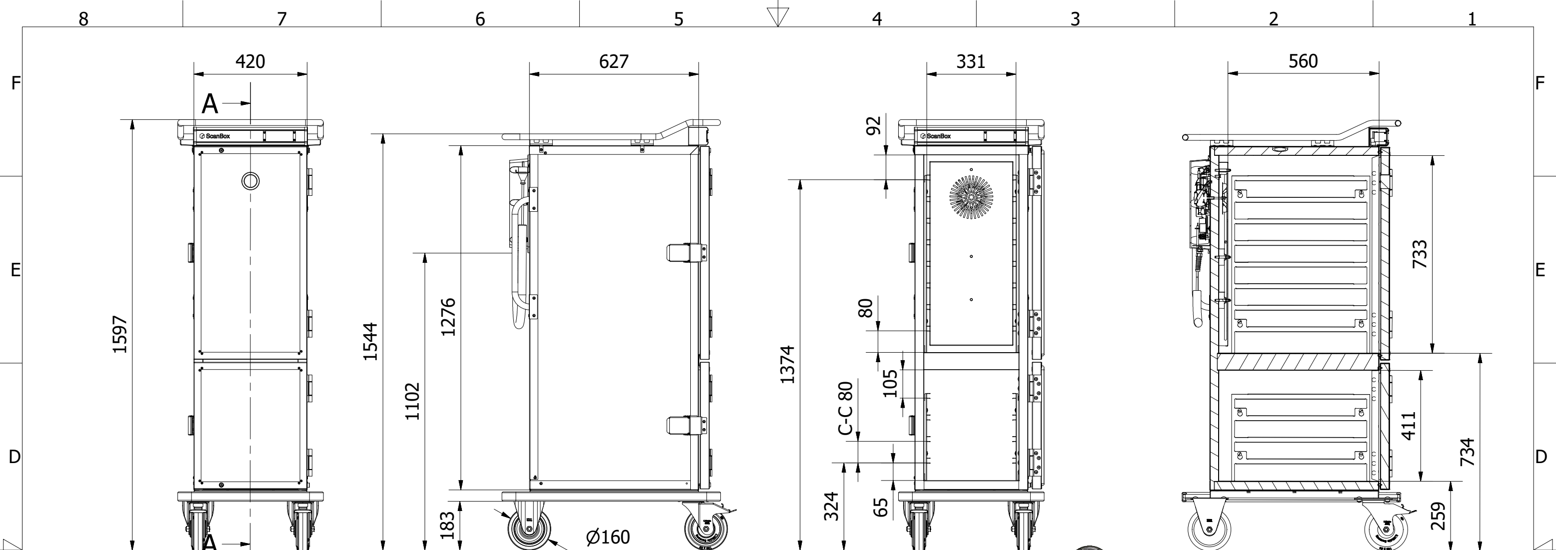
A-A ( 1:14 )
